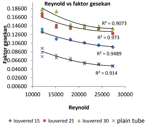
Gambar 6 Grafik perbandingan angka Reynold dengan faktor gesekan berbagai variasi sudut louvered strips
