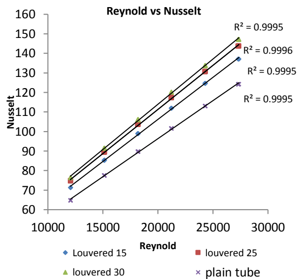
Gambar 5 Grafik perbandingan angka Nusselt dari berbagai variasi sudut louvered strips dengan dengan angka Reynold
