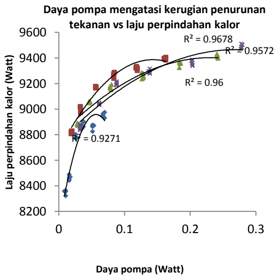
Gambar 10. Grafik perbandingan daya pompa untuk mengatasi kerugian penurunan tekanan dengan laju perpindahan kalor pada berbagai variasi sudut louvered strips
