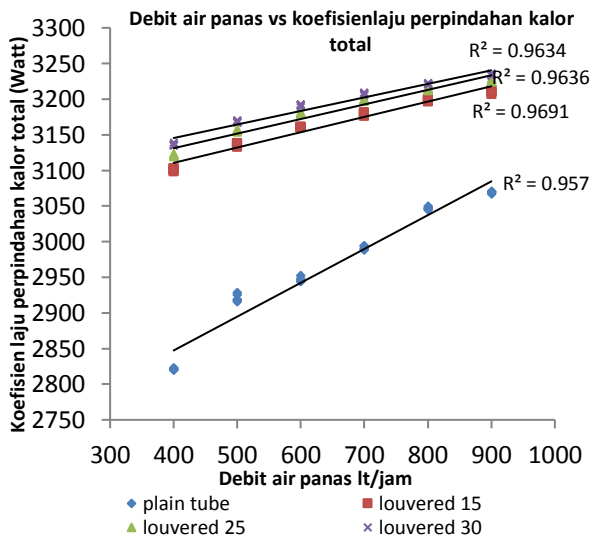
Gambar 7 Grafik perbandingan debit air panas dengan koefisien laju perpindahan kalor total pada berbagai sudut louvered strips
