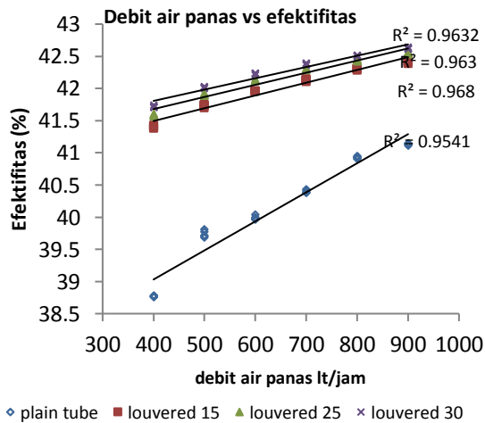
Gambar 9 Grafik pengaruh debit air panas terhadap efektifitas pada tiap-tiap variasi sudut louvered strips
