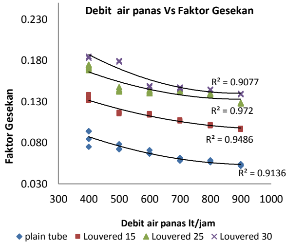
Gambar 3 Grafik pengaruh berbagai variasi sudut louvered strips terhadap faktor gesekan pada berbagai variasi debit air panas
