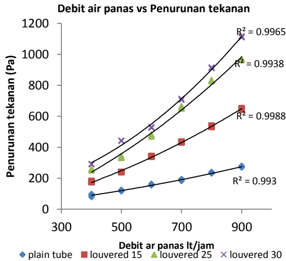
Gambar 8 Hubungan antara variasi debit air panas dengan terhadap penurunan tekanan pada tiap-tiap variasi sudut louvered strips
