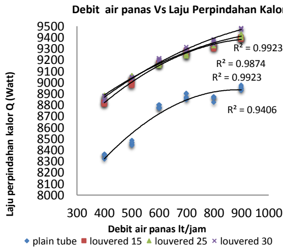
Gambar 4 Grafik pengaruh berbagai variasi sudut louvered strips terhadap laju perpindahan kalor yang ditimbulkan pada berbagai variasi debit
