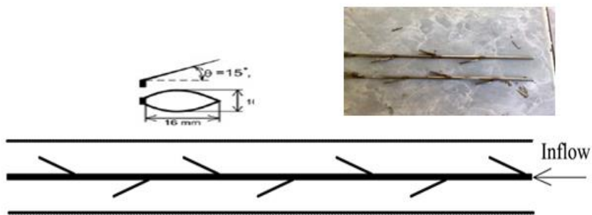
Gambar 2. Ukuran dan bentuk turbulator
