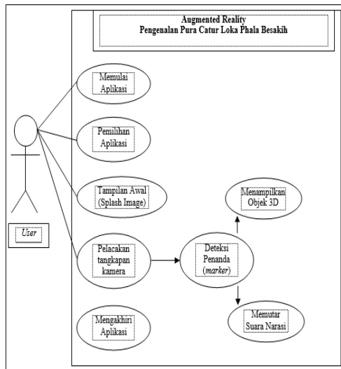
Gambar 4. Use Case Diagram Perangkat Lunak
