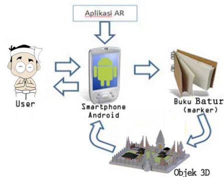
Gambar 2. Blok Diagram Proses interaksi aplikasi dengan user
