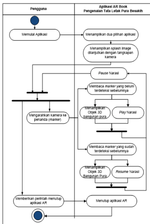
Gambar 5. Activity Diagram Perangkat Lunak
