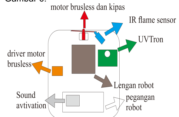
Gambar 6. Lantai 3 robot Penyelamat dan Pemadam Api.
