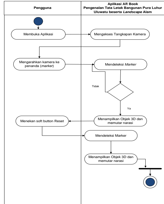
Gambar4d. Activity Diagram Mereset Aplikasi
