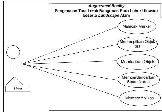
Gambar 3. UseCase Diagram Perangkat Lunak Aplikasi Augmented Reality Book Pengenalan Tata Letak Bangunan Pura Luhur Uluwatu beserta Landscape Alam
