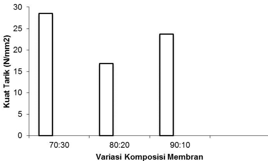
Gambar 4. Hasil kuat tarik membrane.
