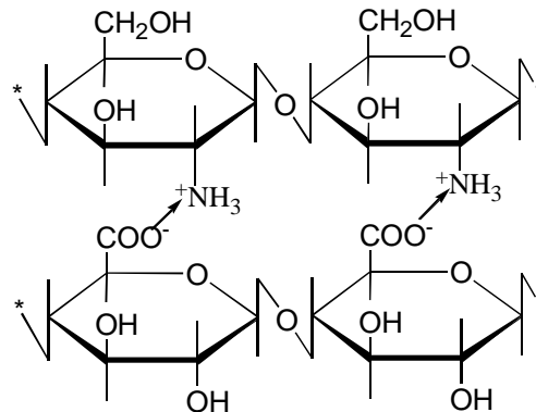
Gambar 2. Struktur hipotetik membran PEC kitosan-pektin
