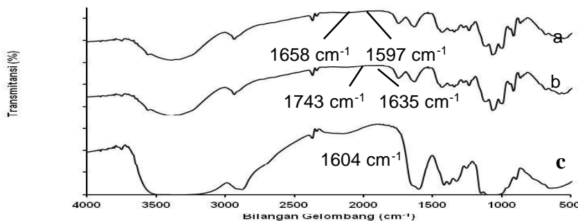
Gambar 1 Spektra IR (a) kitosan, (b)pektin, dan (c) PEC kitosan-pektin
